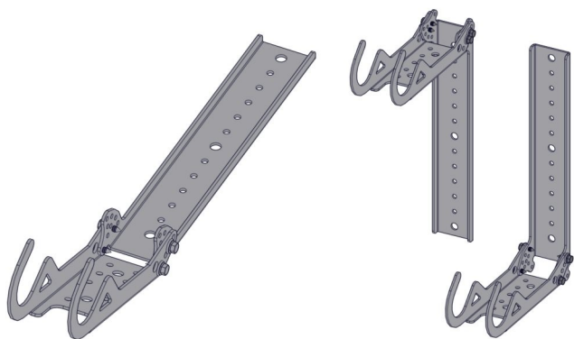
Kroken och fästskenan monteras samman med 4 st självgående skruv 6,3x19 mm.
