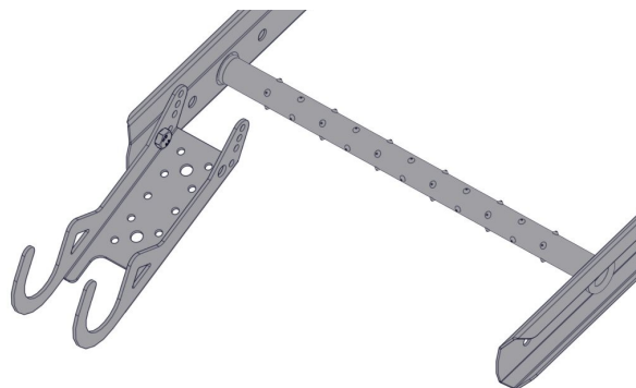
Kroken monteras med bult M10x20 till stegen.
